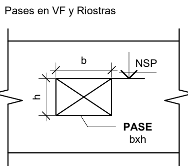
ESQUEMA TIPO
