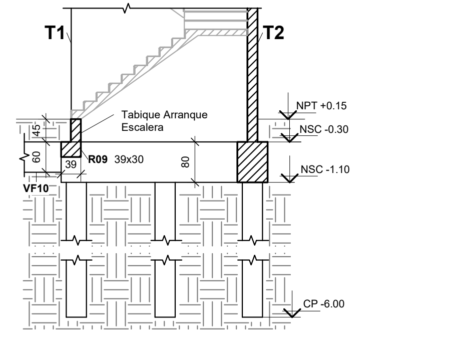
SECCIÓN 2-2
